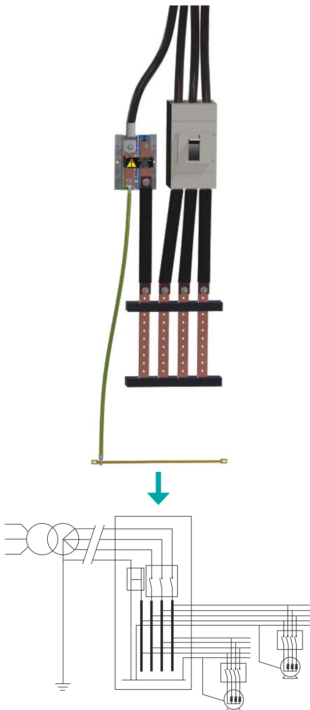
Распределение TN-S
