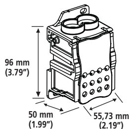
Перемычка UD400J
