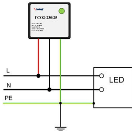
Рис. 1 Подключение ГСО2-230/25
