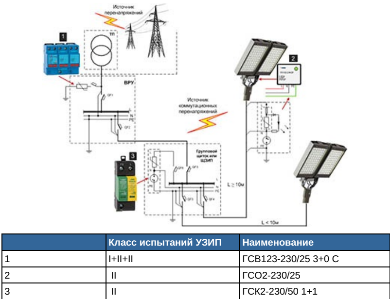
Рис. 3 Пример схемы защиты светодиодных систем для объектов со сложной электромагнитной обстановкой
