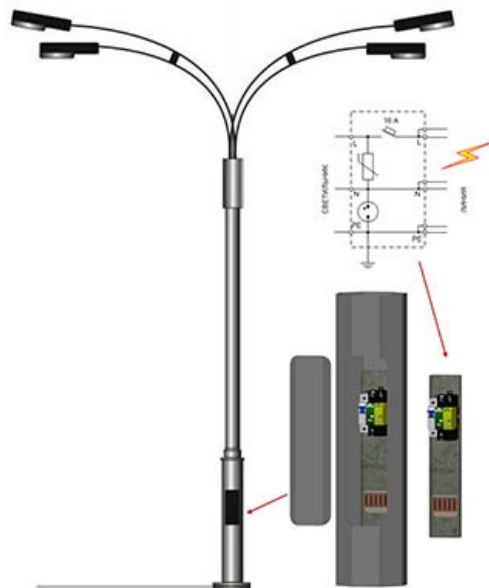
Рис. 4 Размещение ЩЗИП-ОСВ-* в опоре освещения
