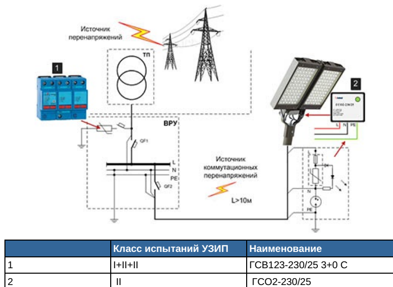
Рис. 2 Пример схемы защиты светодиодных светильников с применением УЗИП непосредственно возле светильника
